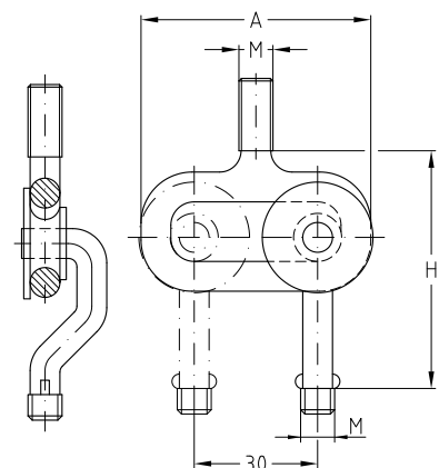
Скользящая скоба в сочетании с хомутом MUPRO
